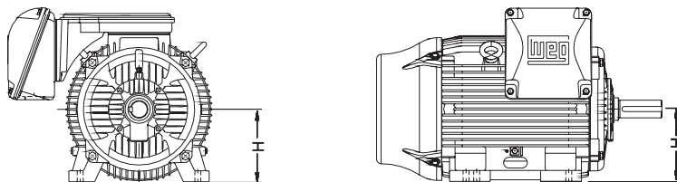
Carcaças 225S/M a 355A/B Figura 3
