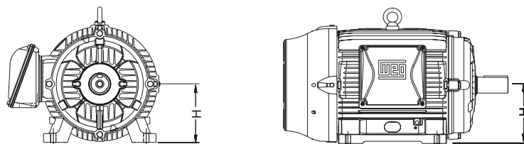
Carcaças 132S a 200L Figura 2
