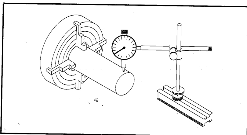
Figura 31 - Verificação da Centralização do Diâmetro Externo de uma Peça Montada na Placa do Torno com o Auxílio de um Relógio Comparador
