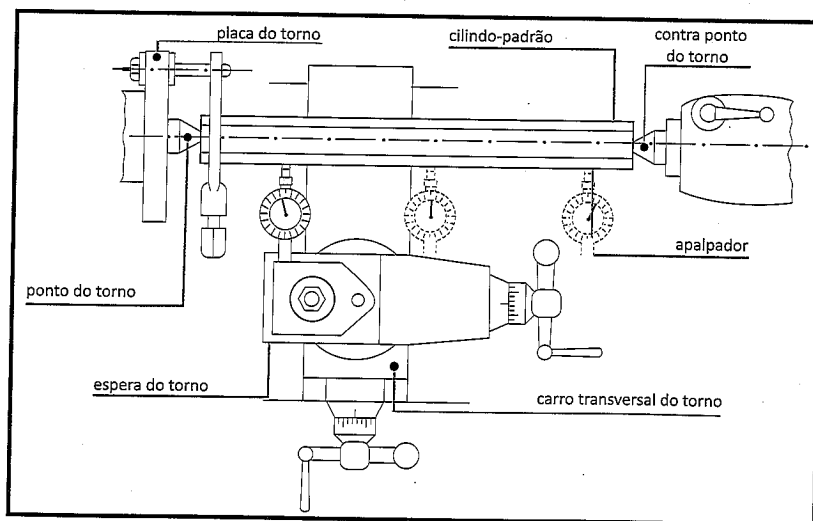
Figura 32 - Verificação do Alinhamento das Pontas de um Torno Mecânico Horizontal com o Auxílio de um Relógio Comparador
