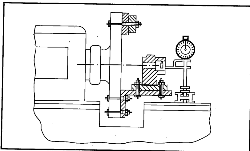
Figura 30 - Verificação da Excentricidade de um Furo de uma Peça Montada na Placa do Torno com o Auxílio de um Relógio Comparador
