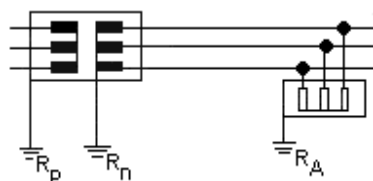
Figura 2 - Esquema TTN
