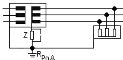
Figura 5 - Esquema ITS
