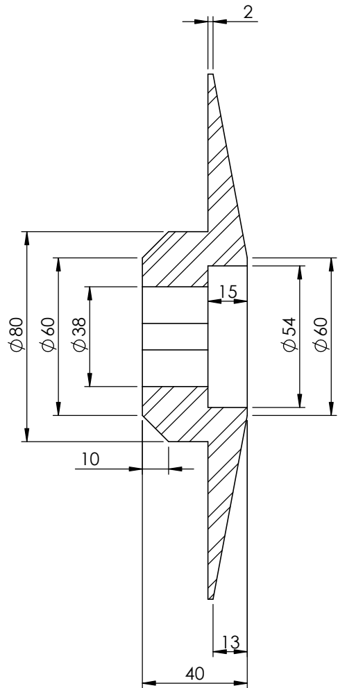
SEÇÃO G-G ESCALA 1 : 2
