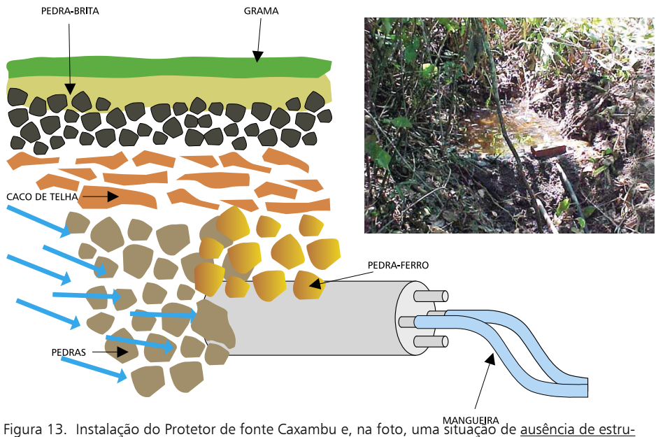
Figura 13. Instalação do Protetor de fonte Caxambu e, na foto, uma situação de ausência de estrutura de proteção.
