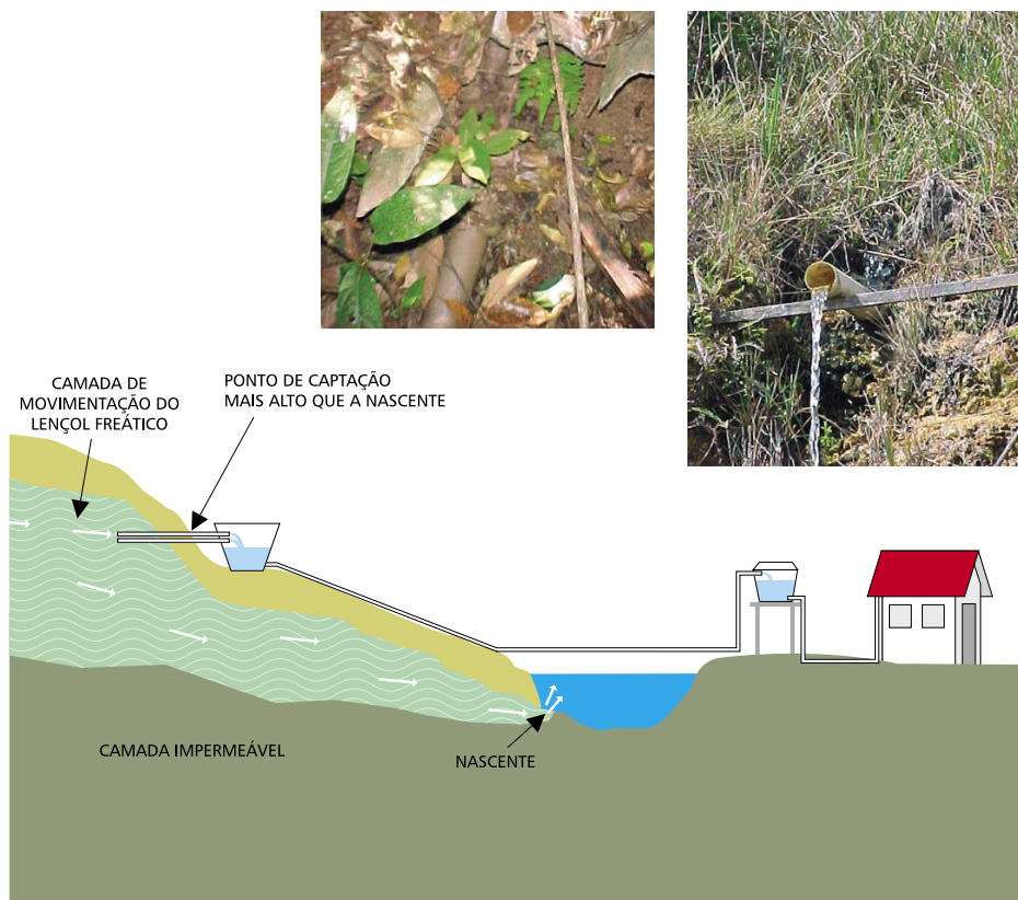
Figura 11. Captação com drenos cobertos. Em detalhe, um dreno saindo da superfície do solo, protegido com uma calha de fibrocimento e um de bica de água potável saindo de um barranco de estrada.
