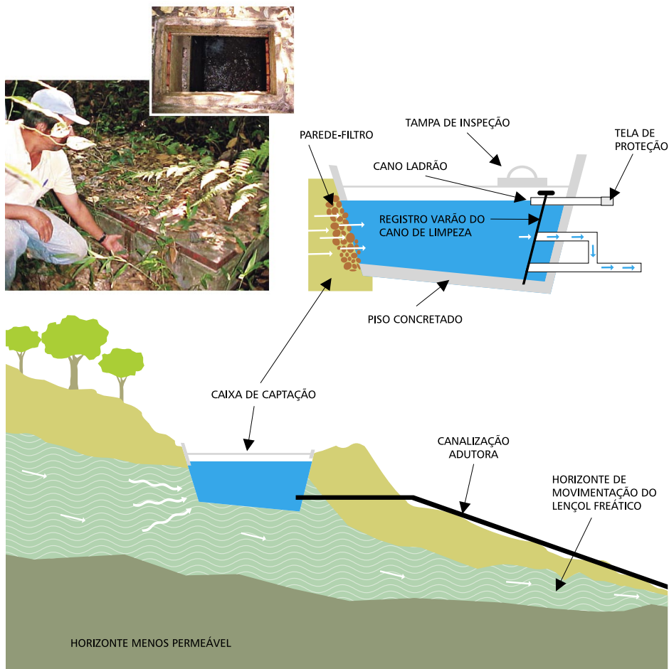
Figura 10. Caixa de proteção de nascente tipo trincheira.
