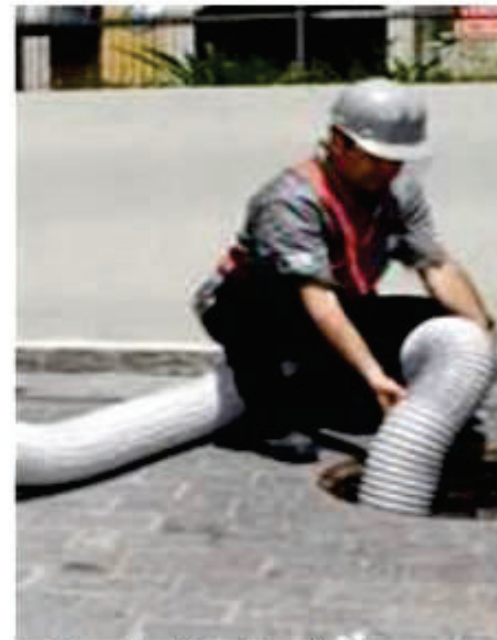
Fig. 5 – Ventilação forçada.
