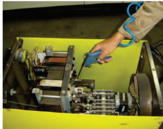
Fig. 43 – Limpeza no interior do equipamento De soldagem, com Ar Comprimido Seco.
