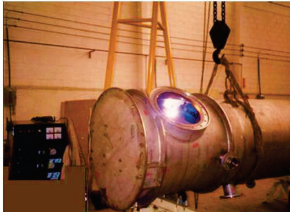
Fig. 53 – Soldagem em ambientes confinados
