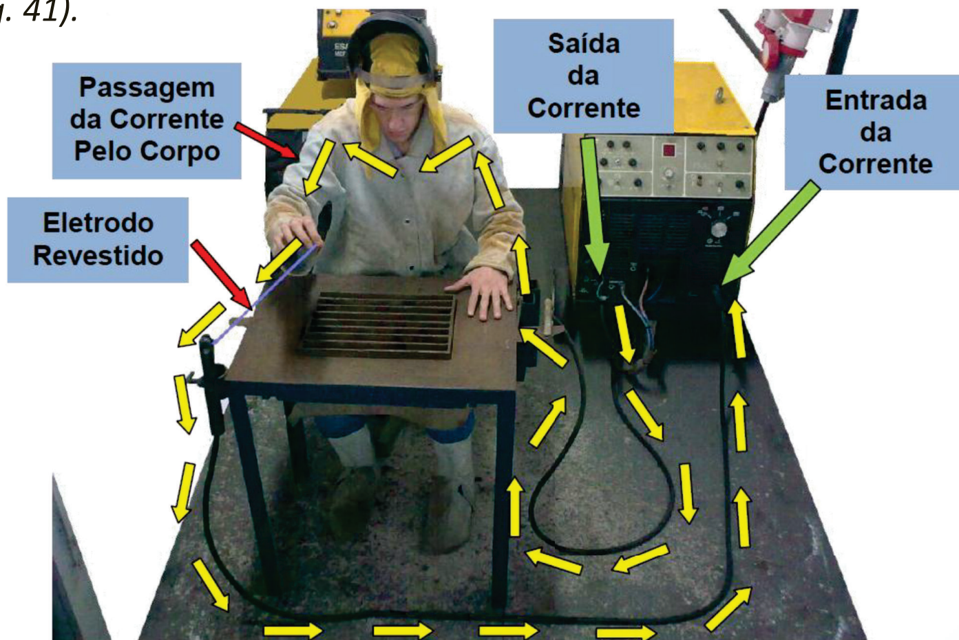
Fig. 41 – Fechamento do Circuito elétrico com o corpo sem luvas
