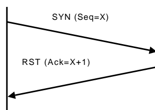
Figura 3.14: Recusa de conexão TCP.
