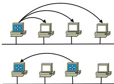
Figura 4.8: Protocolo ARP.
