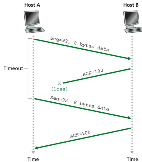
Figura 3.10: Números de sequência TCP: Cenário 1 (KUROSE; ROSS, 2006a).
