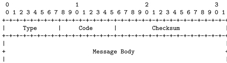
Figura 4.13: Formato geral da mensagem ICMPv6 (RFC2463).
